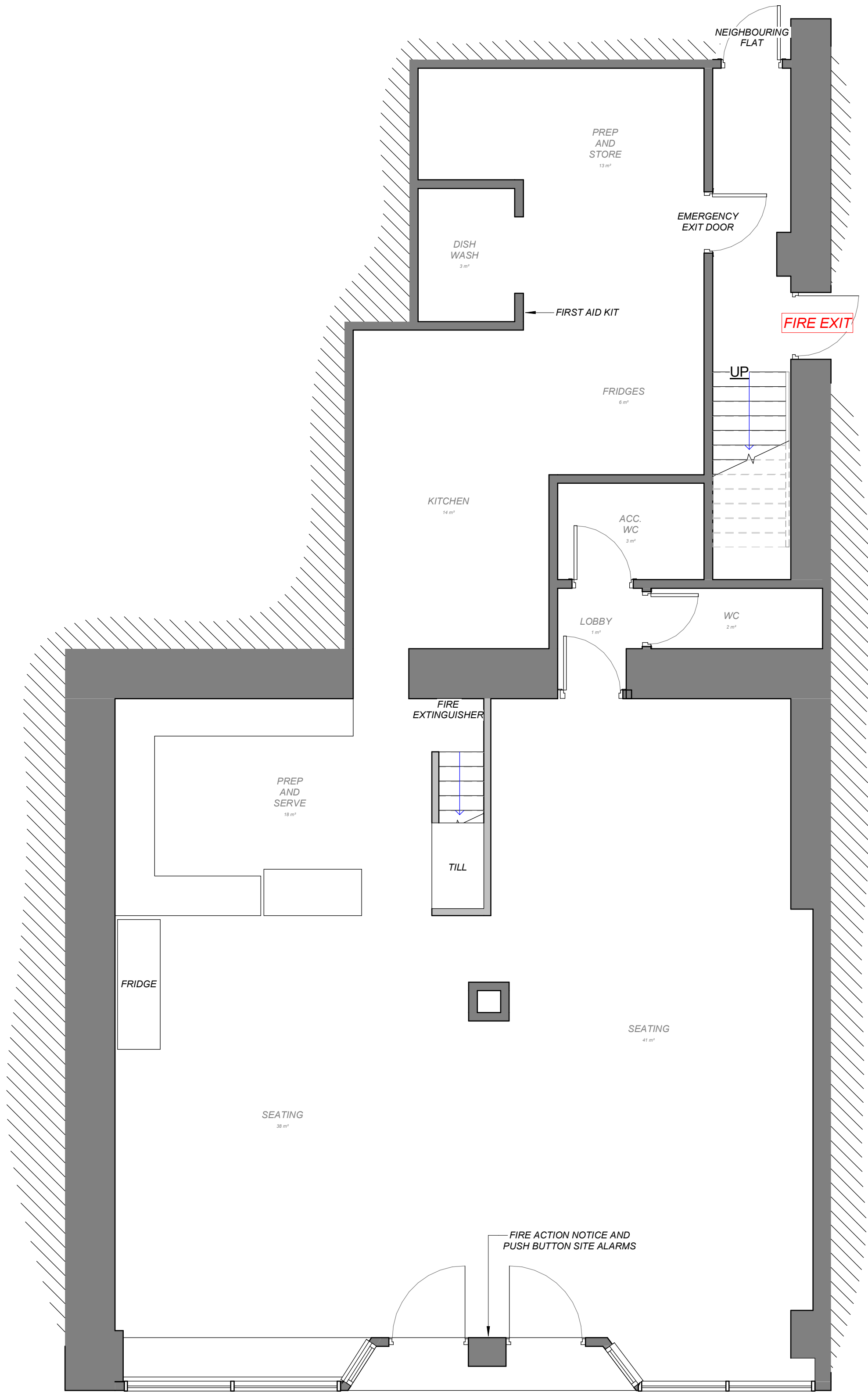
1 01.A1 EXISTING GFL 1 : 50
